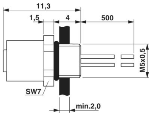
Dessin coté
