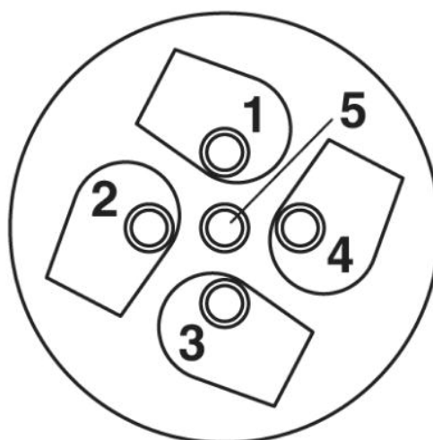
Côté connexion câble M12 (connexion vissée)
