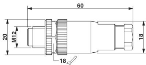
Connecteur mâle M12 x 1, droit
