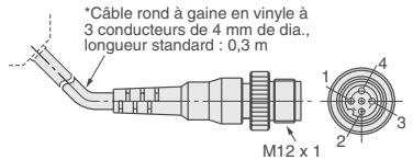
Connecteur précâblé M12 (E3ZM-□□□-M1J)
