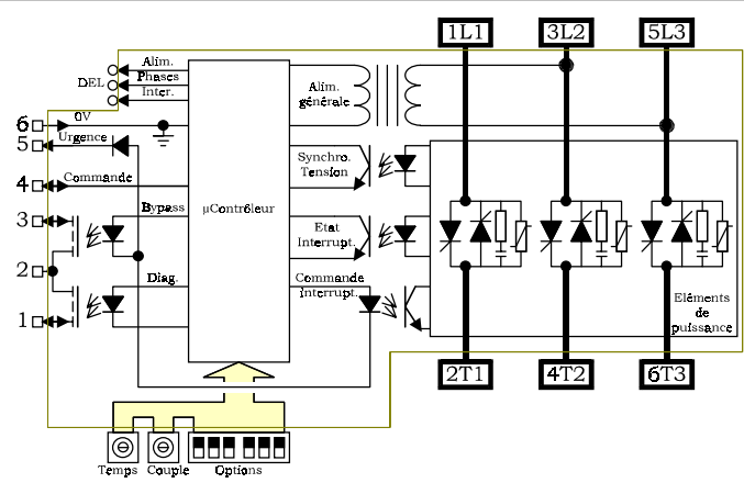
Fig. 1 SYNOPTIQUE INTERNE
